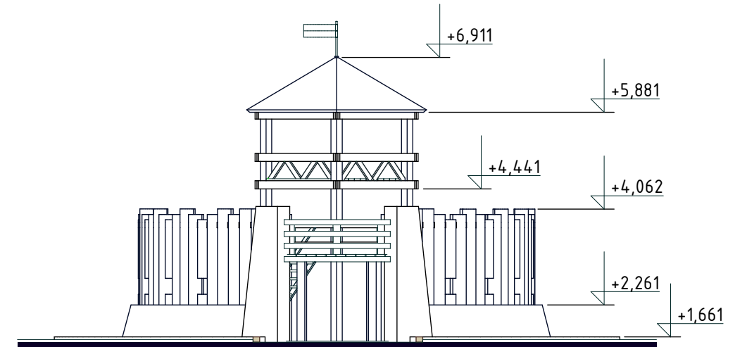
ГОЛОВНИЙ ФАСАД
