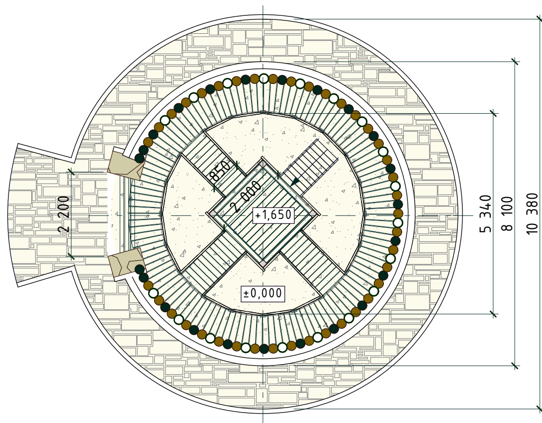
ПЛАН СПОРУДИ
